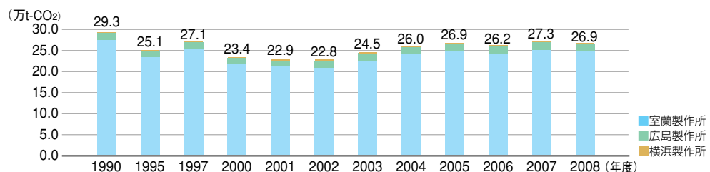
二酸化炭素排出量の推移
