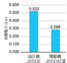
製品1shotあたりの消費電力比較 (650T)
