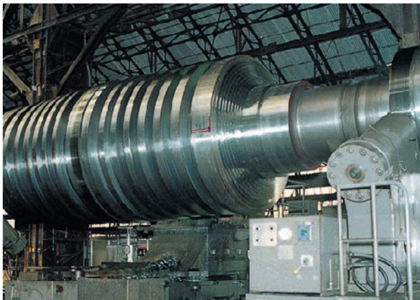
発電用一体型ロータシャフト
